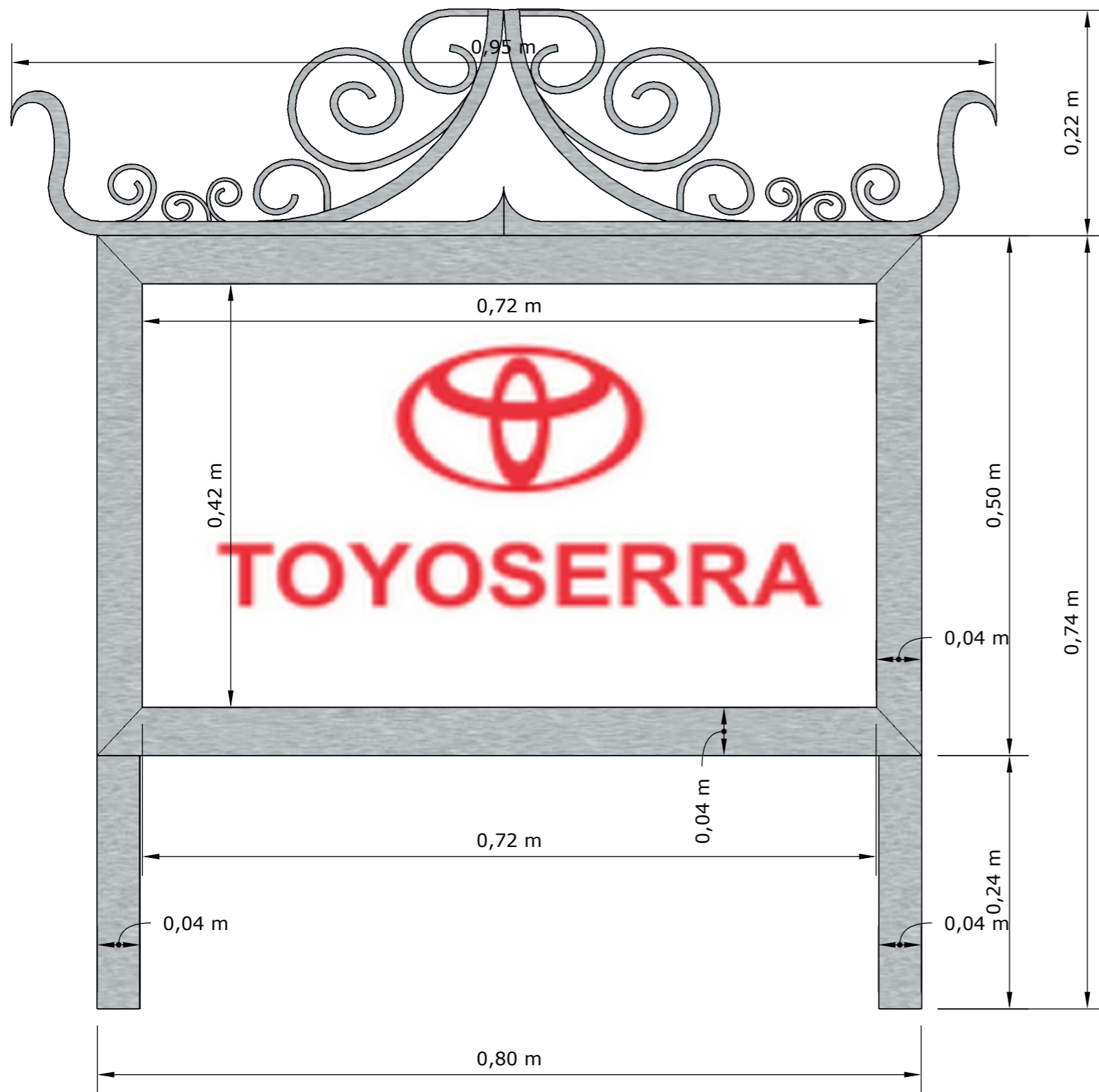
1 VISTA FRONTAL 1/5
