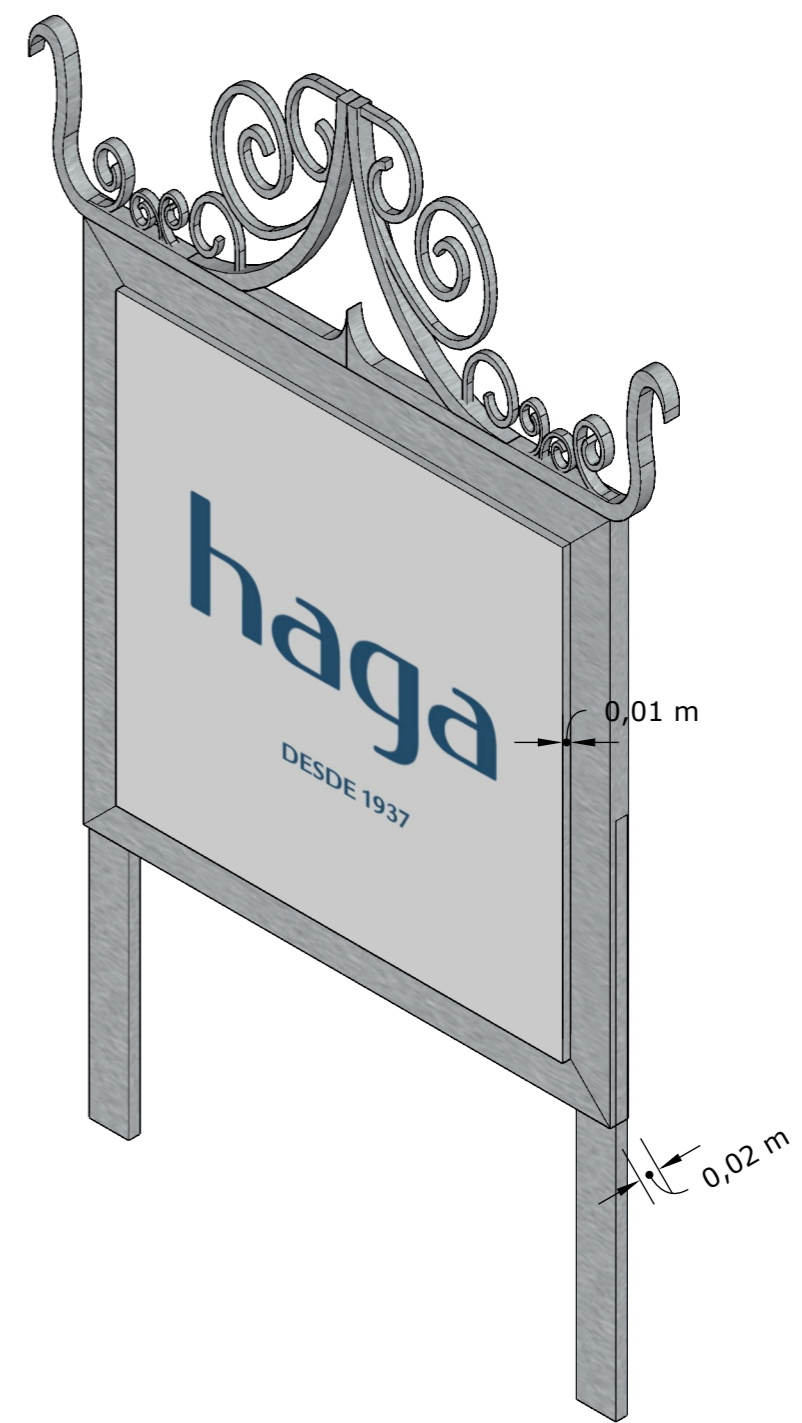
1 PERSPECTIVA ISOMÉTRICA 1/5
