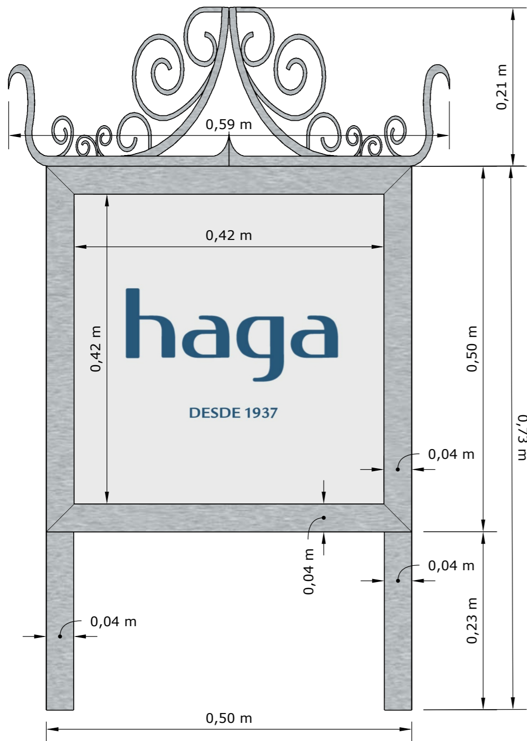
1 VISTA FRONTAL 1/5
